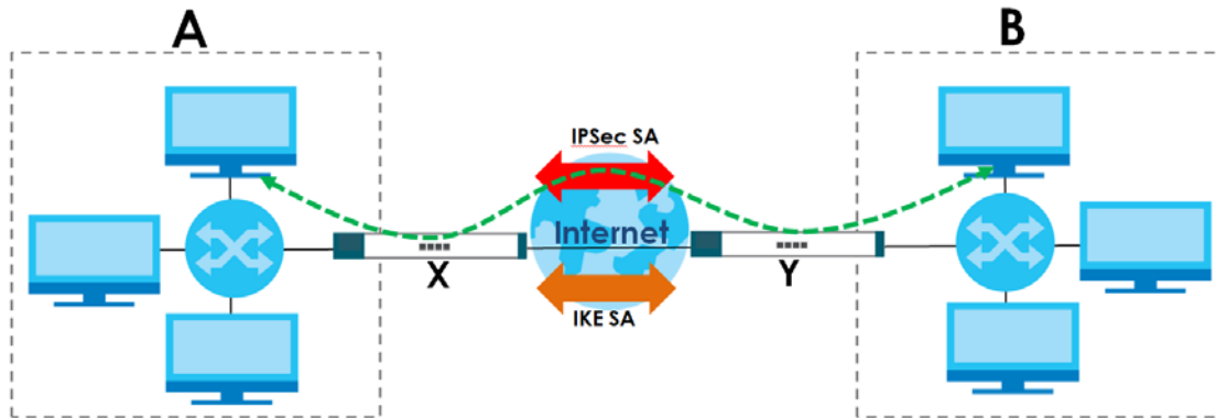
Figure 245 VPN: IKE SA and IPsec SA
